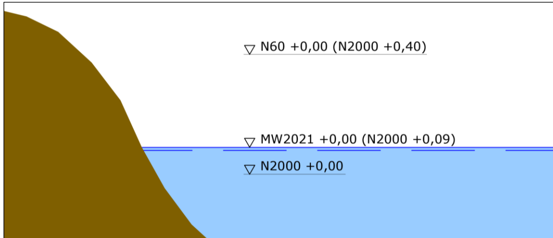
Kuva 6. Periaatekuva vedenkorkeudesta eri korkeusjärjestelmissä Oulussa vuonna 2021.
