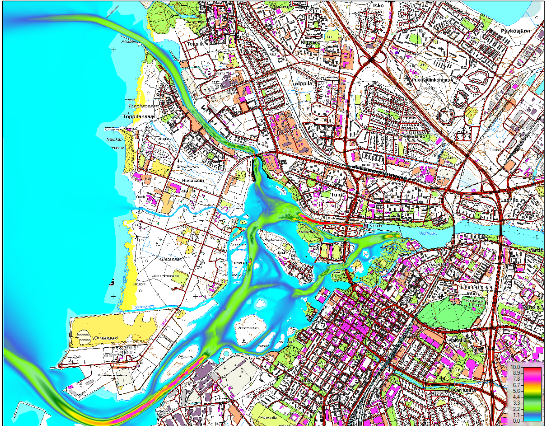
Kuva 22. Virtausnopeus*vesisyvyys [ \text{m}^2/\text{s} ] mallinnustapauksessa 2C1: ylivirtaama HQ_M ja keskialivesi MNW, nykytila (topografia C1). Vesisyvyydellä kerrottu virtausnopeus kuvaa virtaamaa paremmin kuin pelkkä virtausnopeus.
