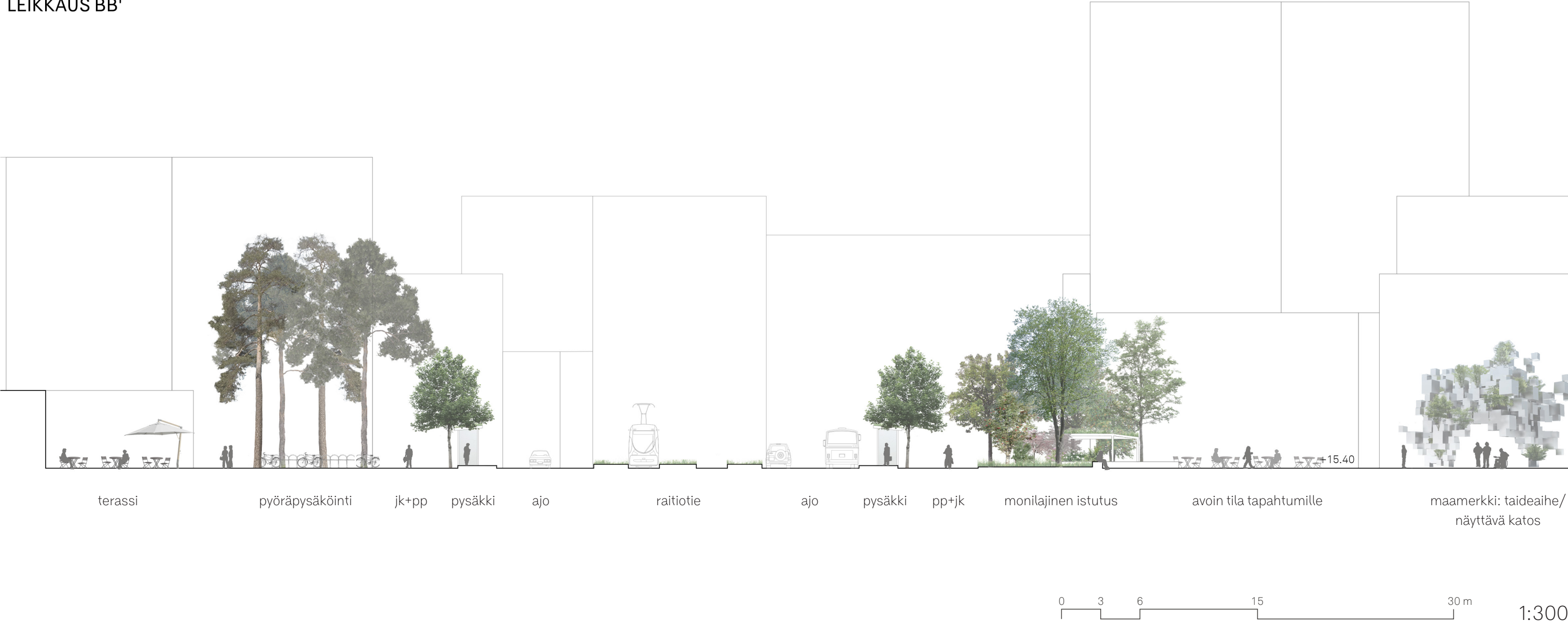
LEIKKAUS BB'
