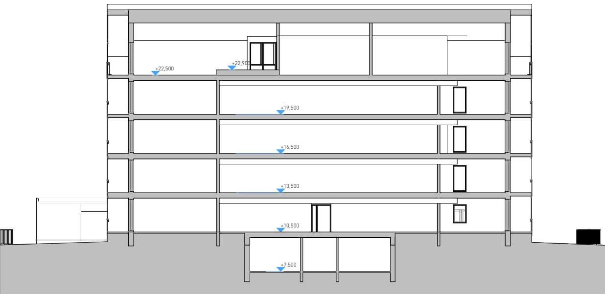
Leikkaus
