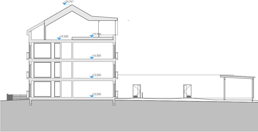
Leikkaus
