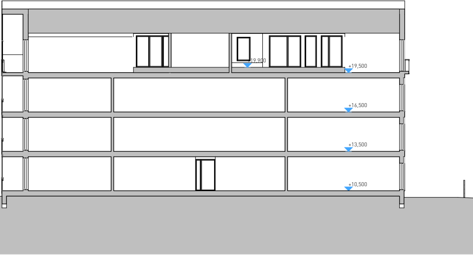
Leikkaus
