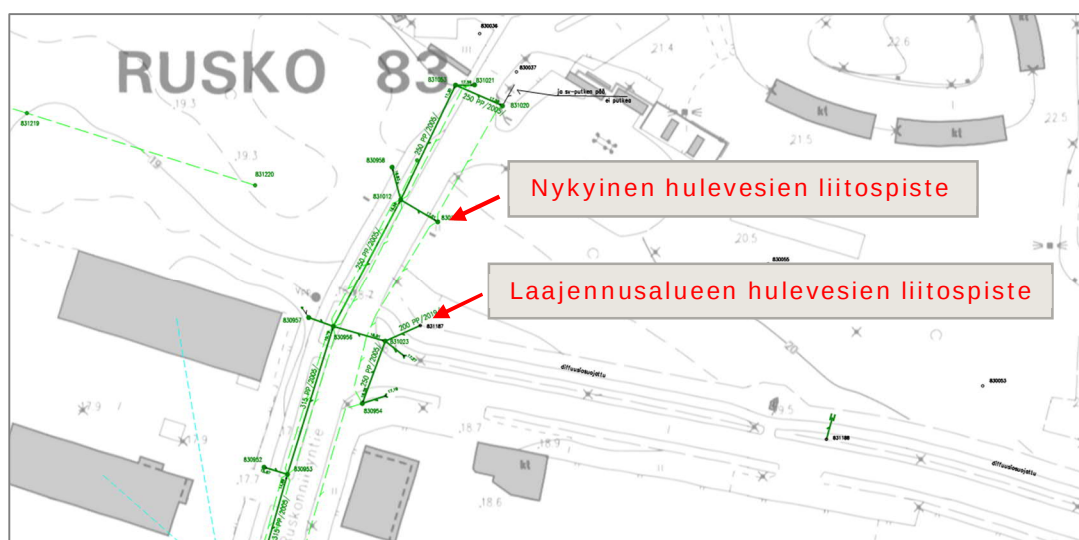
Kuva 8. Hulevesien liittospisteet. (Oulun kaupunki, muokannut Eija Toivonen)
