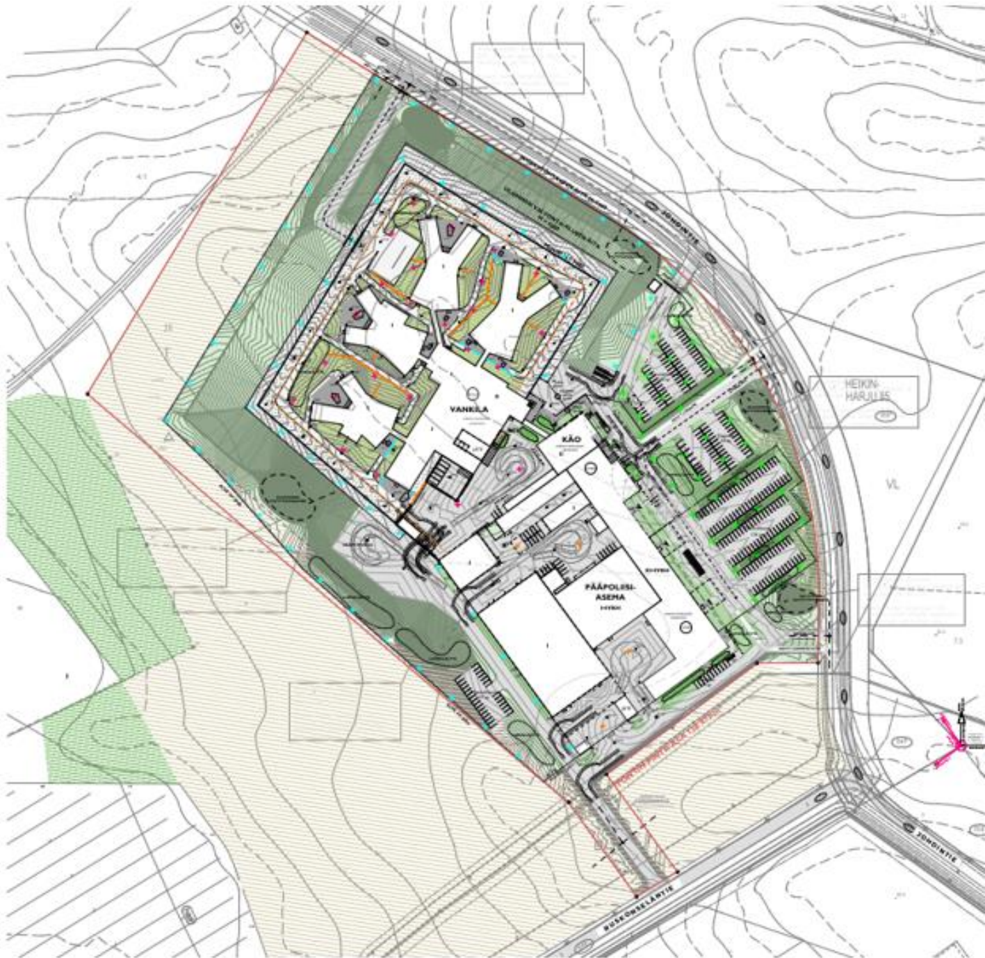
kuva 26, vankilan ja poliisilaitoksen alustava tontinkäyttösuunnitelma 4.5.2022
