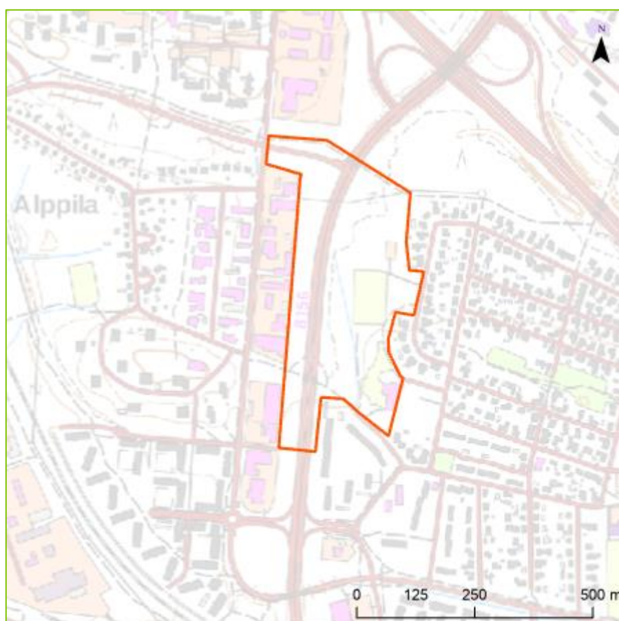
Kuva 2. Selvitysalueen raja.
