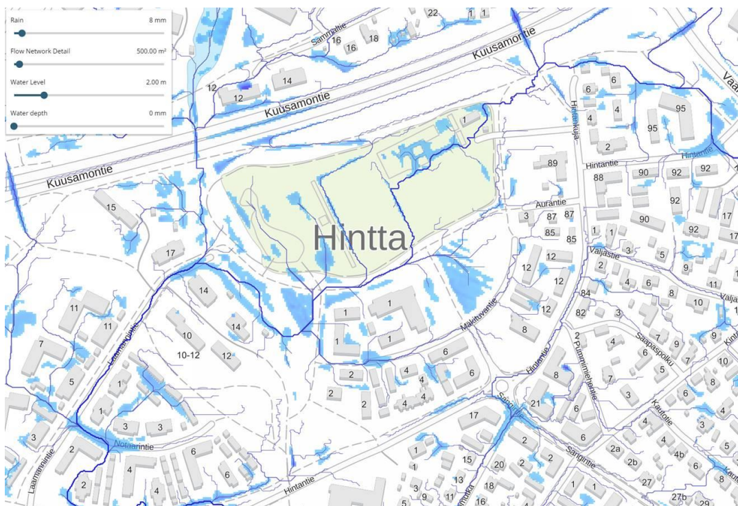
Kuva 6. Alueen tulvareitit
