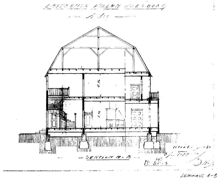
Leikkauspiirustus 1930-luvulta ja oikealla alkuperäinen leikkaus
